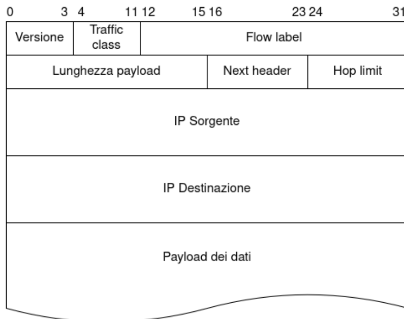
Figura 4.7: Intestazione IPv6
